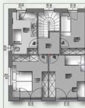
OBERGESCHOSS 58,95m 2
