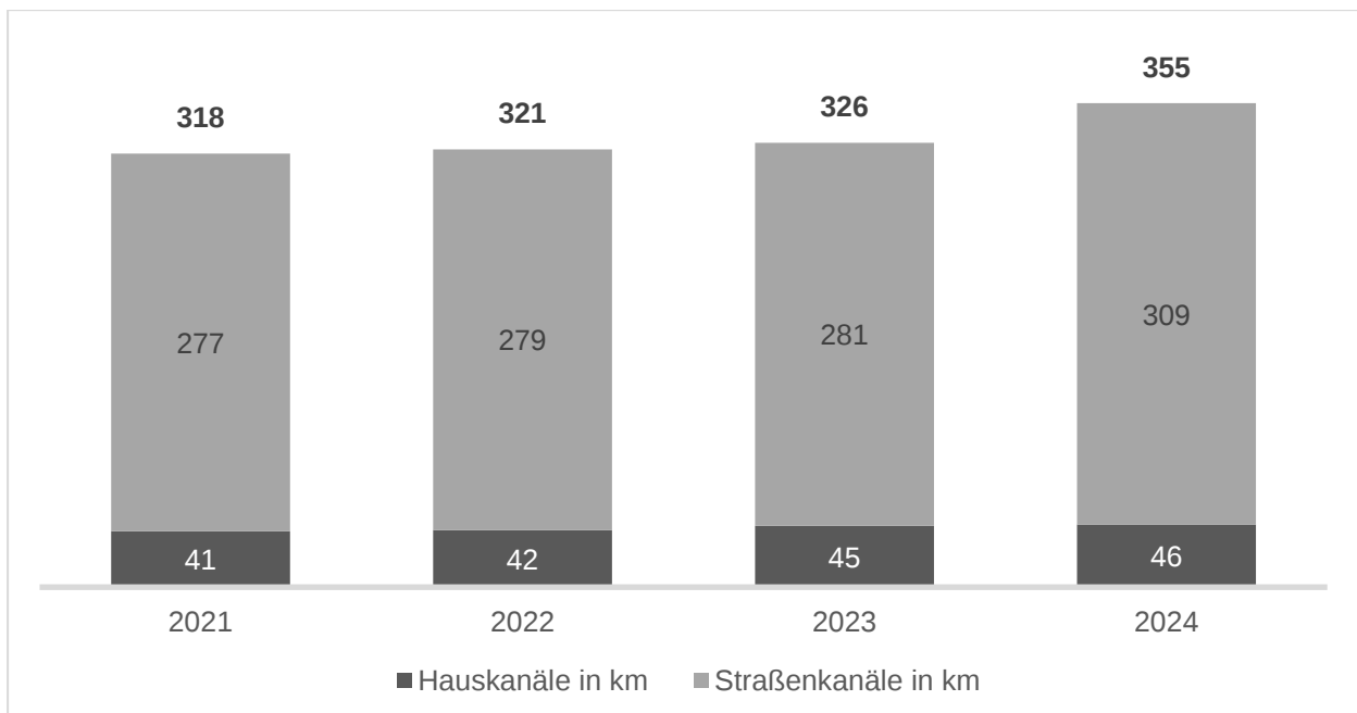
Diagramm 35: Kanalnetz
