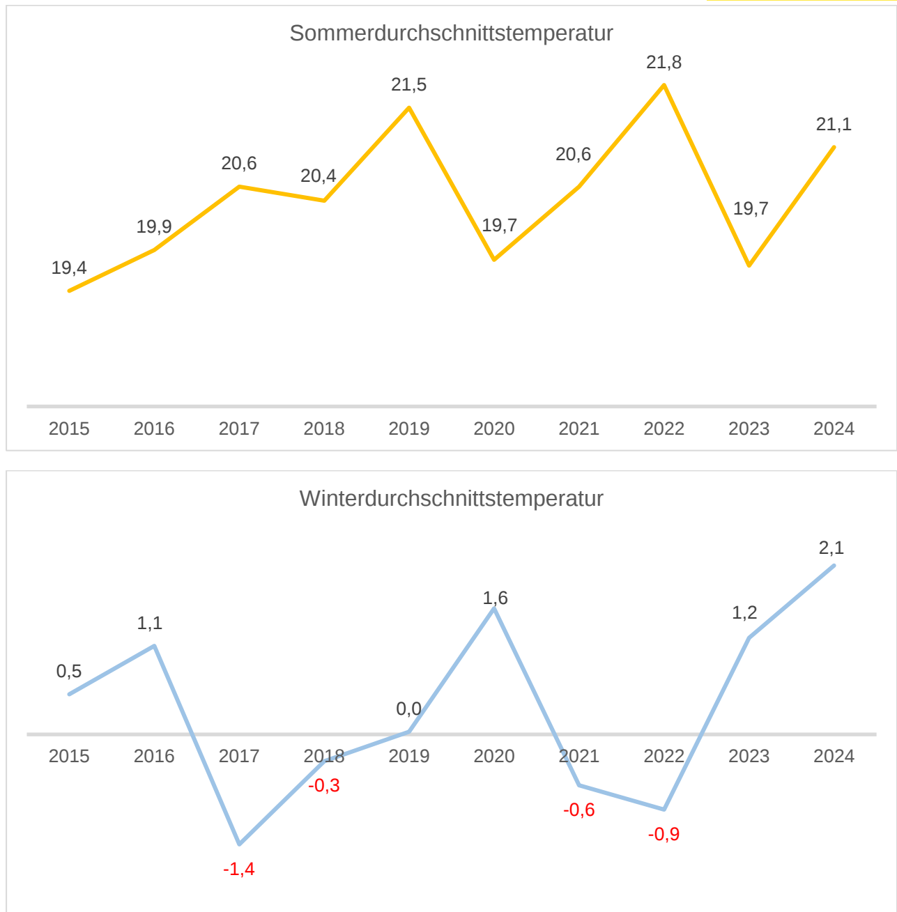
Diagramm 1: Temperaturverläufe
