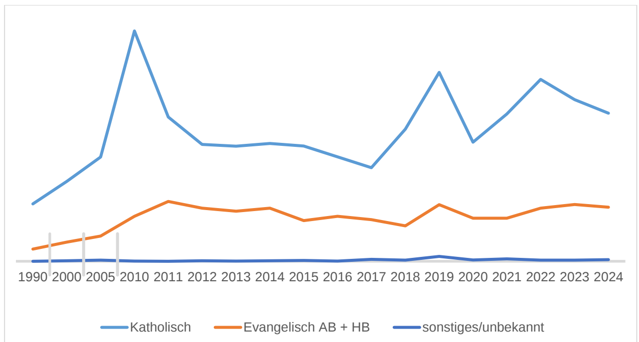
Diagramm 16: Kirchengaustritte
