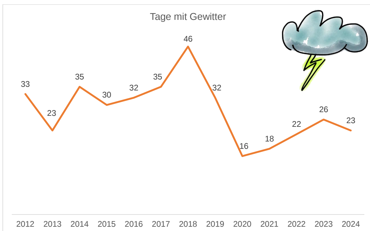
Diagramm 7: Tage mit Gewitter
