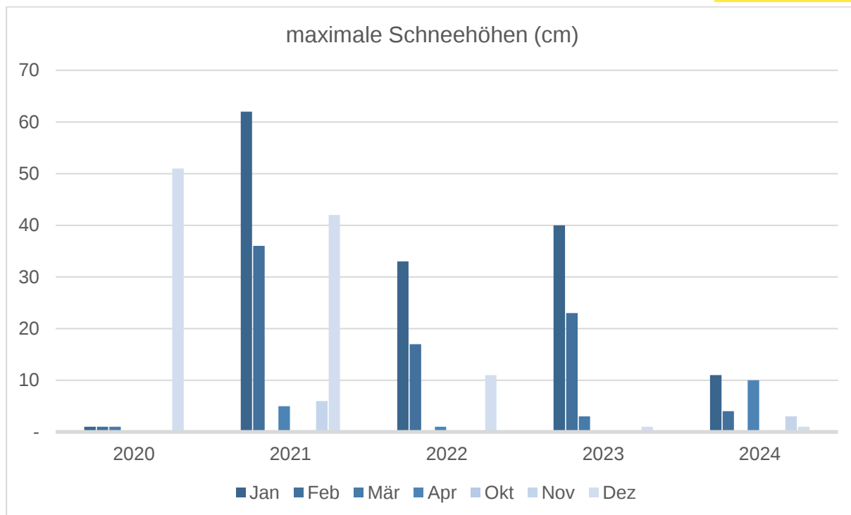
Diagramm 6: maximale Schneehöhen
