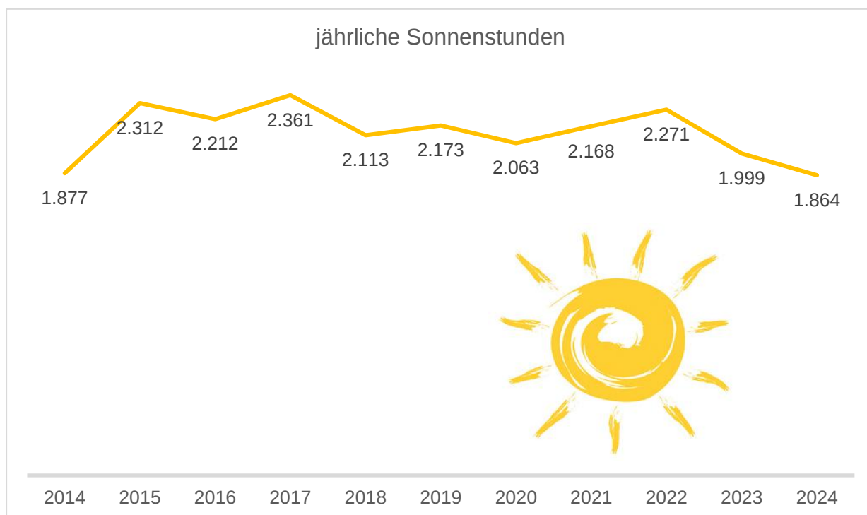
Diagramm 8: Sonnenstunden
