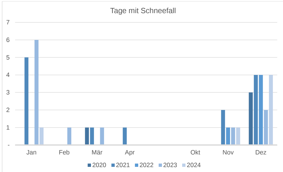
Diagramm 5: Tage mit Schneefall
