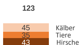
Diagramm 22: Wildabschüsse
