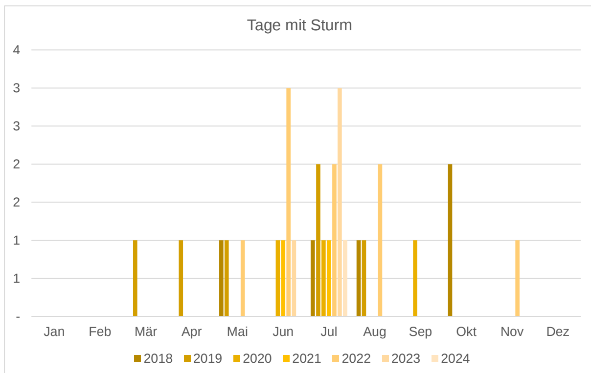
Diagramm 3: Sturmtage
