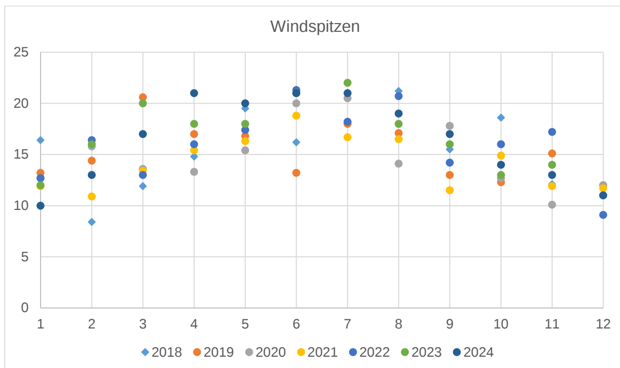
Diagramm 2: Windspitzen
