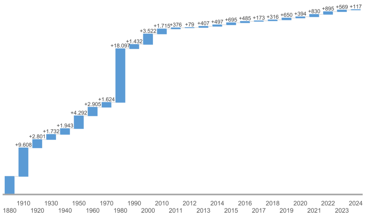
Diagramm 9: Bevölkerungsentwicklung
